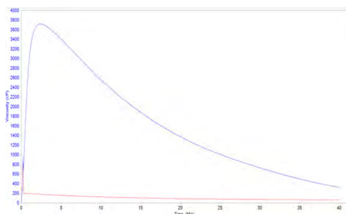
Fig.1 Curva de viscosidad de la disolución de HydroStar en electrolito de cobre en función del tiempo a 120°F.
