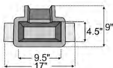
5" PROFUNDIDAD (6" EXTERNA)
